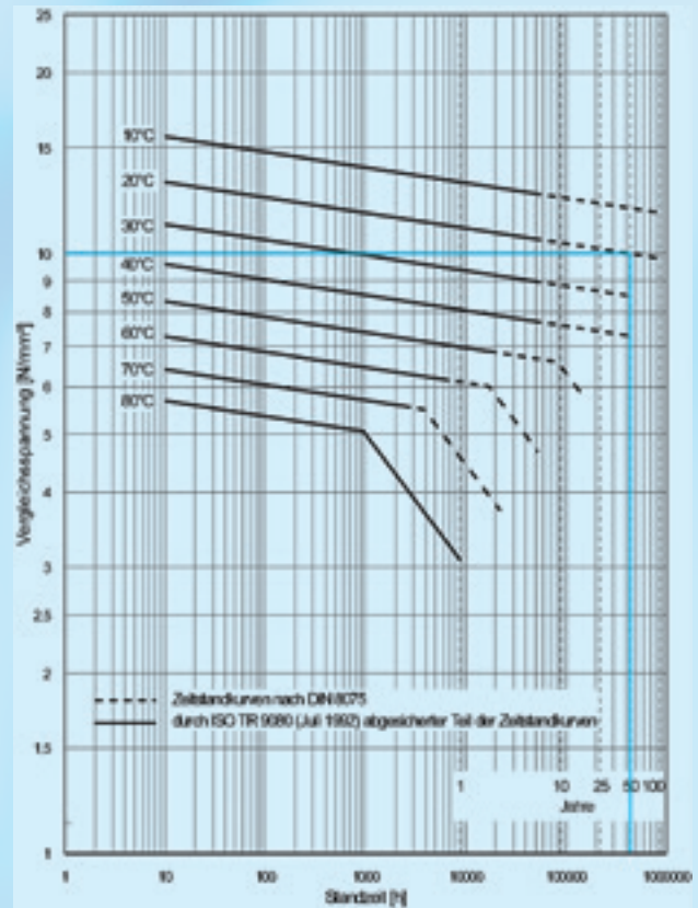
Anforderungen an ein PE 100, dargestellt anhand der Zeitstandfestigkeitskurven der DVS 2205 Teil 1. Bei einer Einsatztemperatur von 20 °C sollte ein PE 100 über eine Lebensdauer von 50 Jahren eine Mindestfestigkeit von 10 N/mm 2 behalten.
