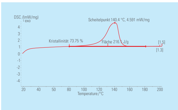
Typisches Diagramm einer DSC-Analyse
