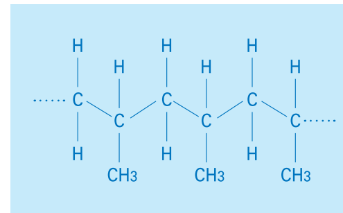
Molekularstruktur eines isotaktischen Polypropylens
