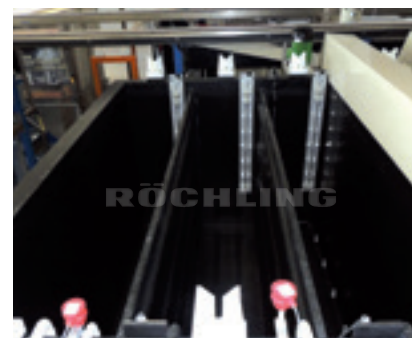
Behälter aus Polystone® G HD schwarz in einer Galvanikanlage
