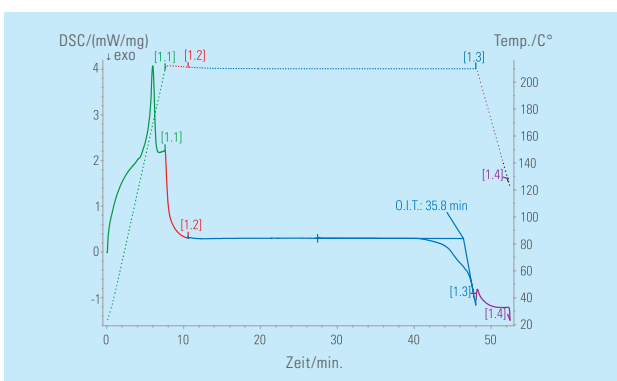
Typisches Diagramm einer OIT-Analyse
