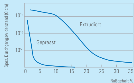
Spez. Durchgangswiderstand in Abhängigkeit von der Rußkonzentration
