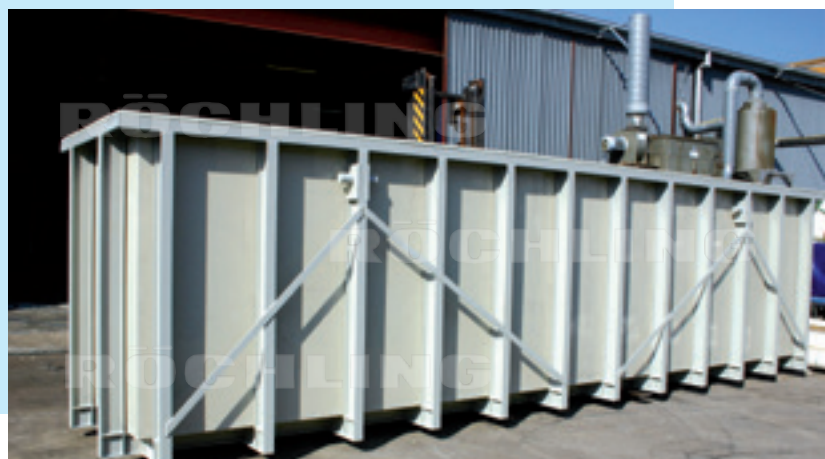
Mit RITA® 4 berechneter Rechteckbehälter mit Jochverstärkung
