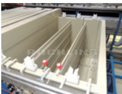
Polystone® P Homopolymer grau Prozessbehälter in einer Kunststoffgalvanik
