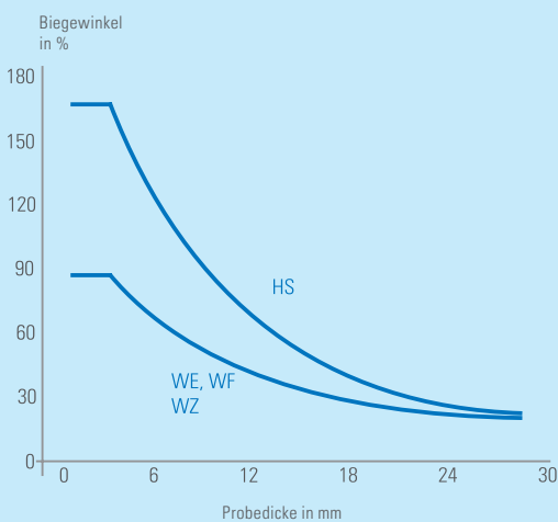
Mindestbiegewinkel für PE-HD (PE 80, PE 100) gemäß DVS 2203-1 Beiblatt 3
