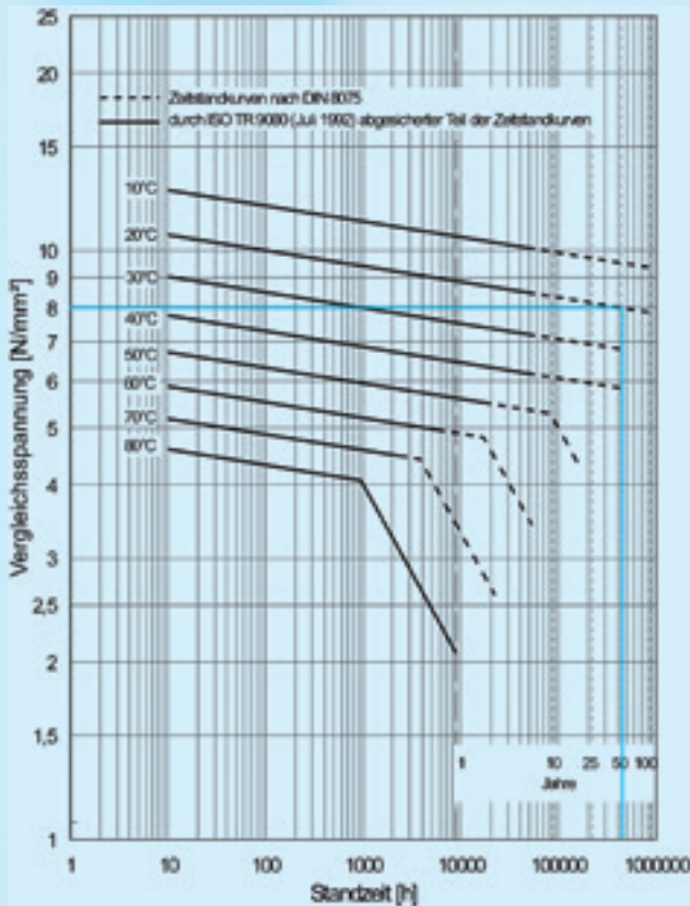
Anforderungen an ein PE 80, dargestellt anhand der Zeitstandfestigkeitskurven der DVS 2205 Teil 1. Bei einer Einsatztemperatur von 20 °C sollte ein PE 80 über eine Lebensdauer von 50 Jahren eine Mindestfestigkeit von 8 N/mm 2 behalten.
