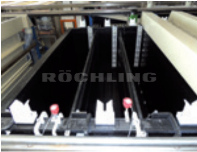
Polystone® G HD schwarz Prozessbehälter in einer Kunststoffgalvanik
